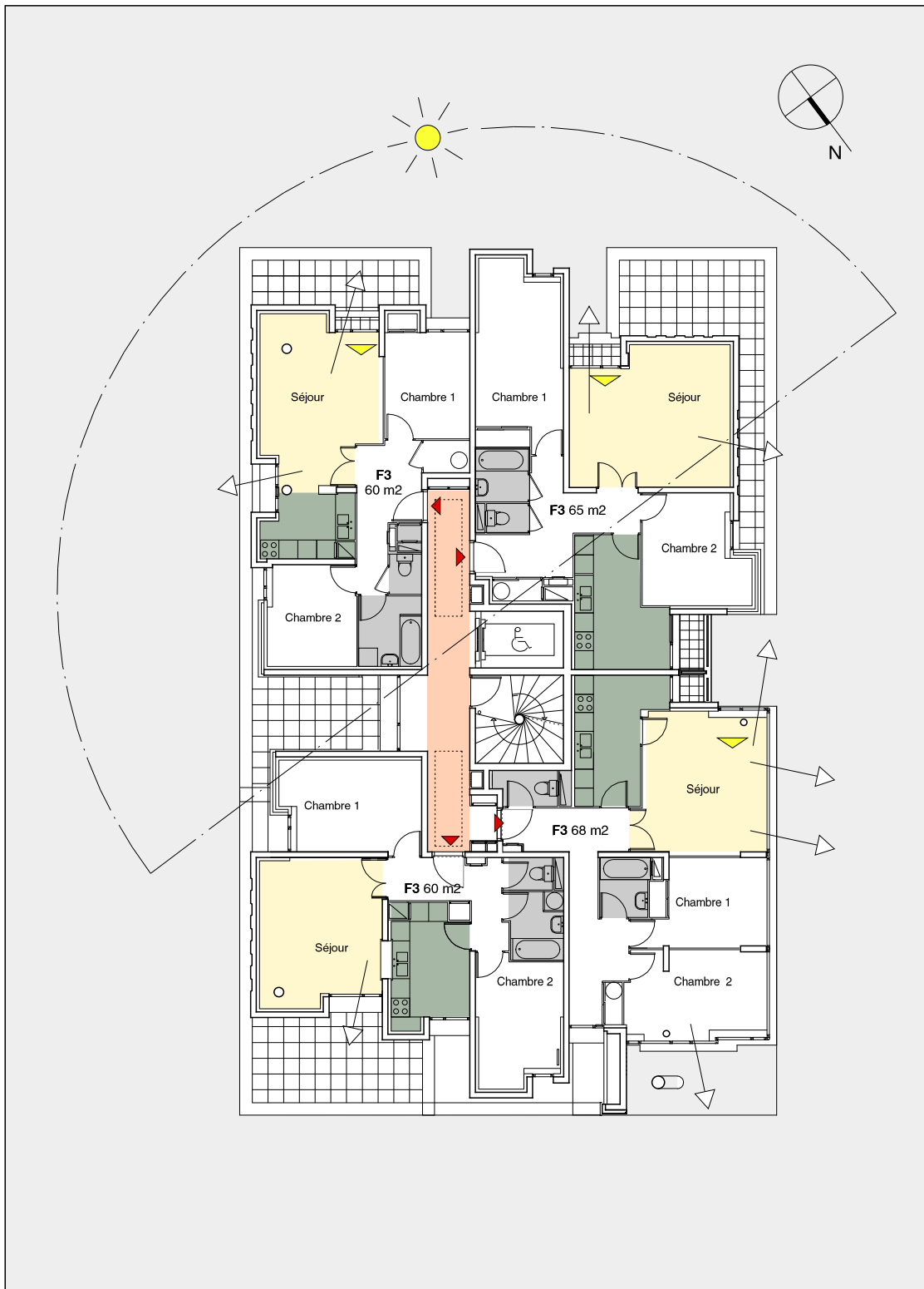
PLAN D'ETAGE COURANT (R+6)
